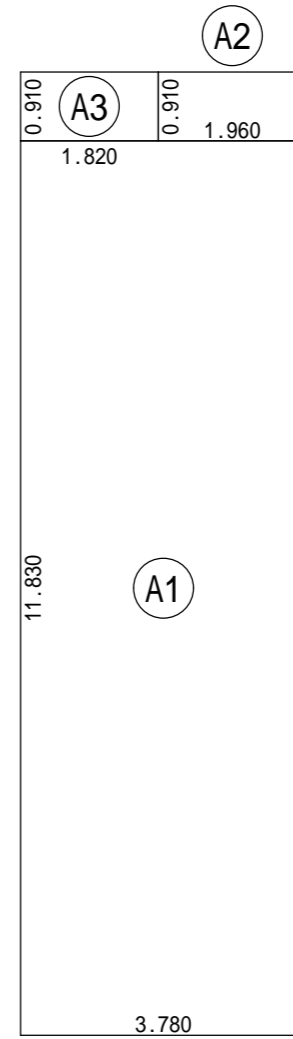
2階 床面積求積図 S:1/100
